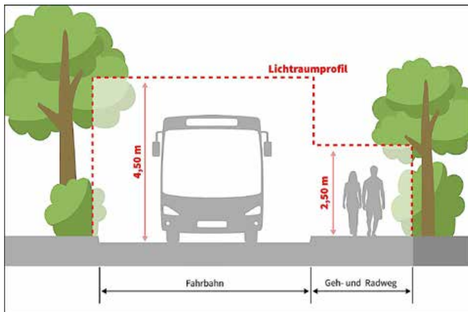
Schematische Darstellung des Lichtraumprofils.
